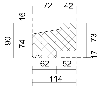
Kozijnhout 90 x 114 mm
