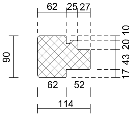
Kozijnhout 90 x 114 mm
