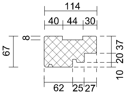
Kozijnhout 67 x 114 mm
