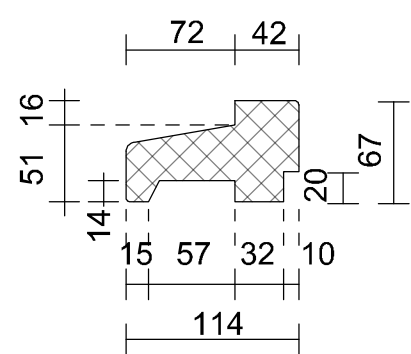
Kozijnhout 67 x 114 mm
