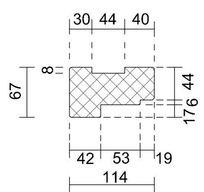
Kozijnhout 67 x 114 mm
