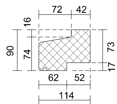
Kozijnhout 90 x 114 mm
