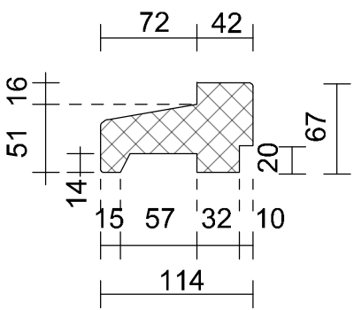
Kozijnhout 67 x 114 mm
