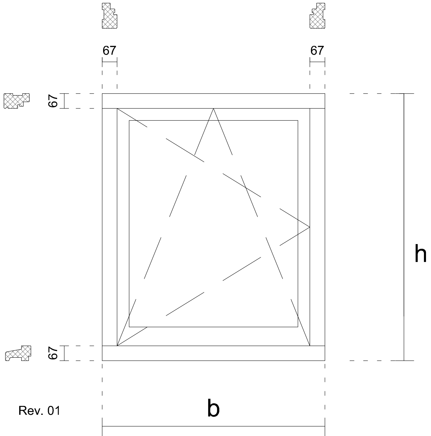
Kozijnhout 67 x 114 mm
