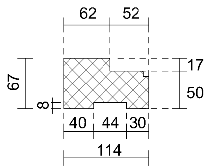
Kozijnhout 67 x 114 mm
