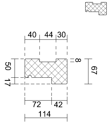
Kozijnhout 67 x 114 mm
