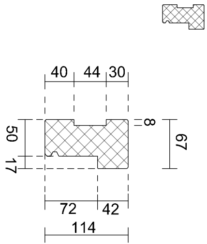
Kozijnhout 67 x 114 mm
